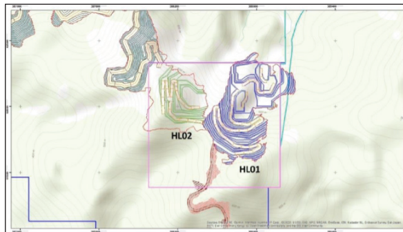
Desain Pit HL01 dan HL02
